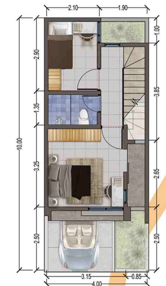
LANTAI 2
