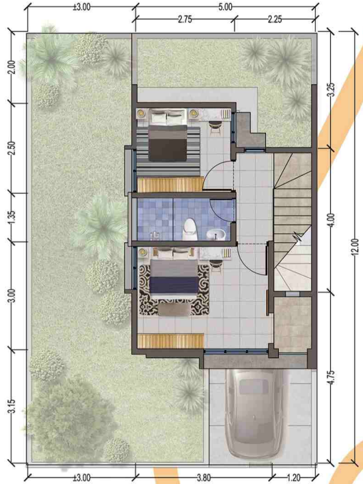
LANTAI 2
