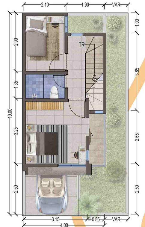
LANTAI 2
